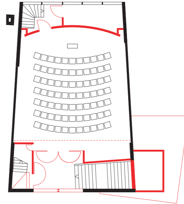
DACHGESCHOSS
